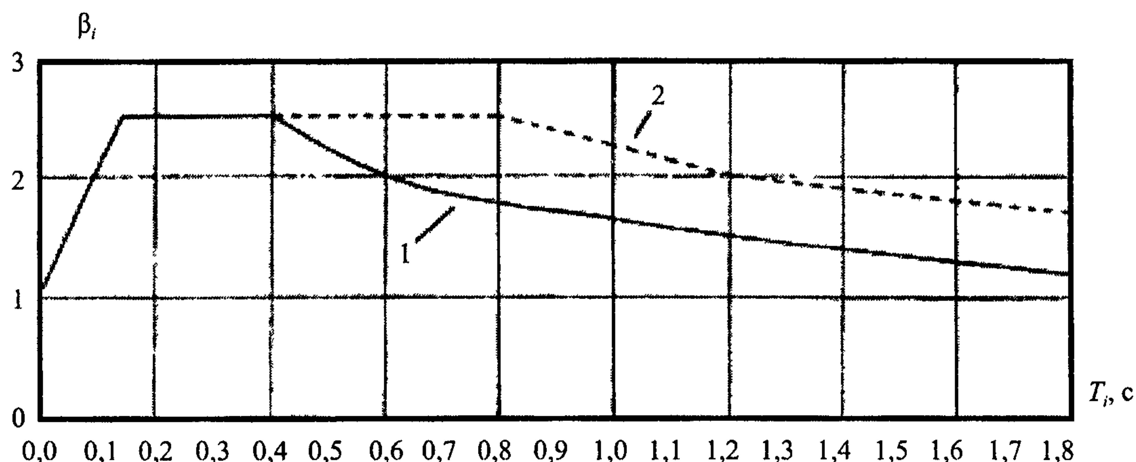
Рисунок 3 – Коэффициенты динамичности \beta(T_i)
